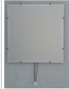
OA Model
